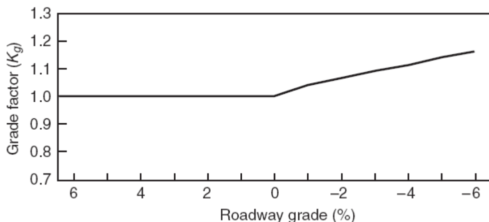
Σχήμα 2: Συσχέτιση K_g με την κατά μήκος κλίση της σήραγγας [6]
